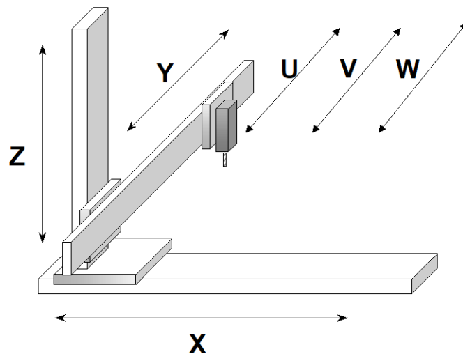
Figure 2.2.1 三軸直角正交(X-Y-Z)，外加三軸輔助軸(U、V、W)
