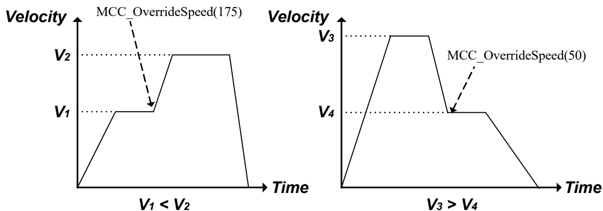
Figure 2.6.4 速度強制
