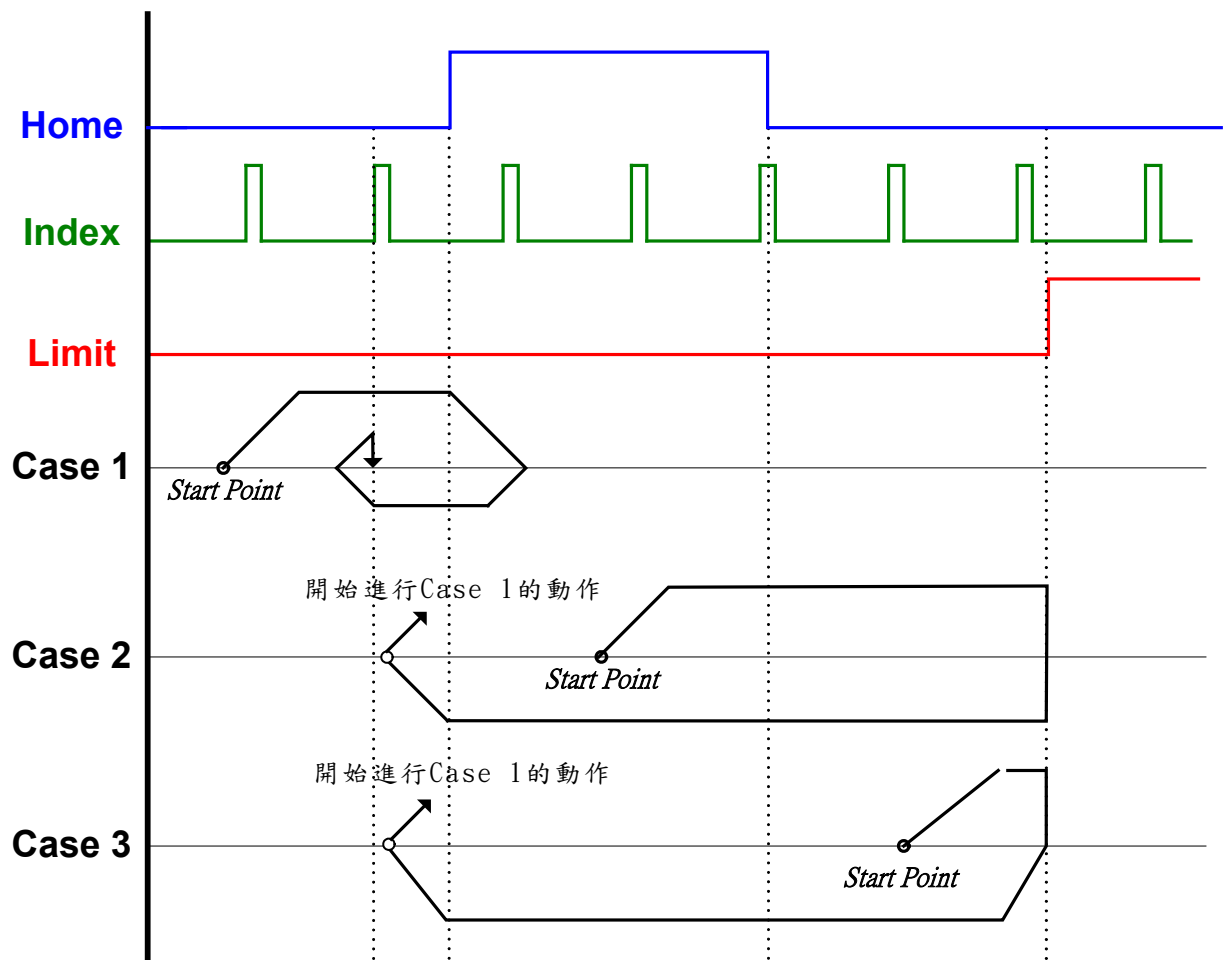
Figure 2.8.1 不同起始點對原點復歸動作的影響
