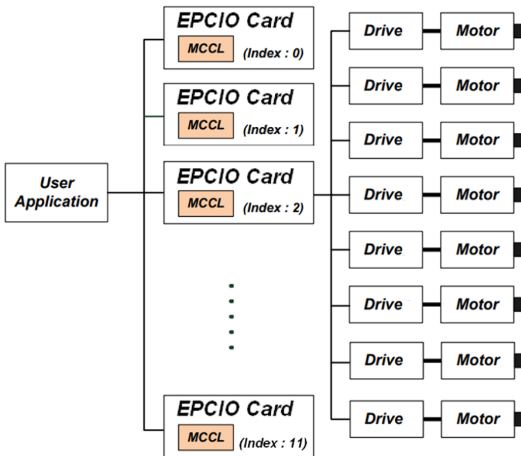
Figure 2.2.2 MCCL 可搭配 12 張 EPCIO 卡
