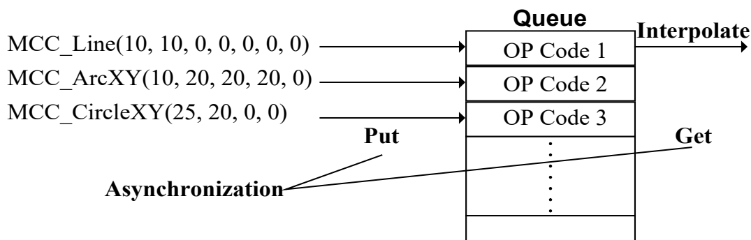
Figure 2.3.2 運動命令緩衝區
