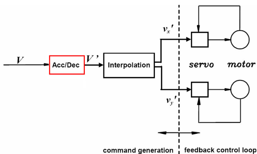
Figure 2.6.7 前加減速模式插值流程
