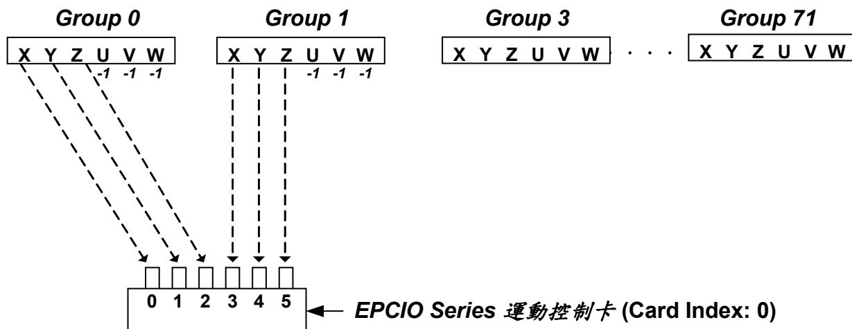
Figure 2.4.5 Group 參數設定
