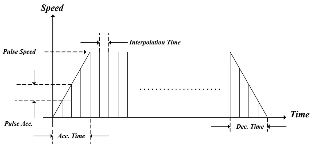
Figure 2.6.5 軌跡規劃設定參數
