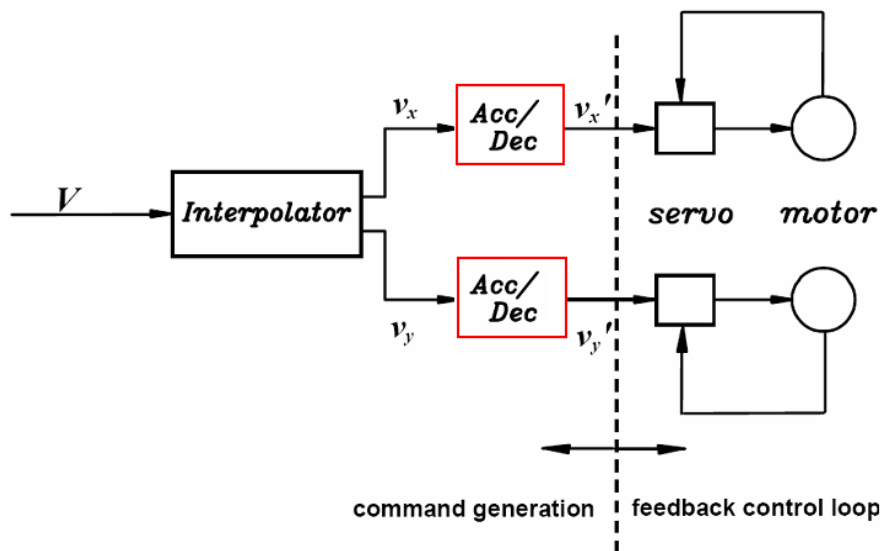
Figure 2.6.6 後加減速模式插值流程
